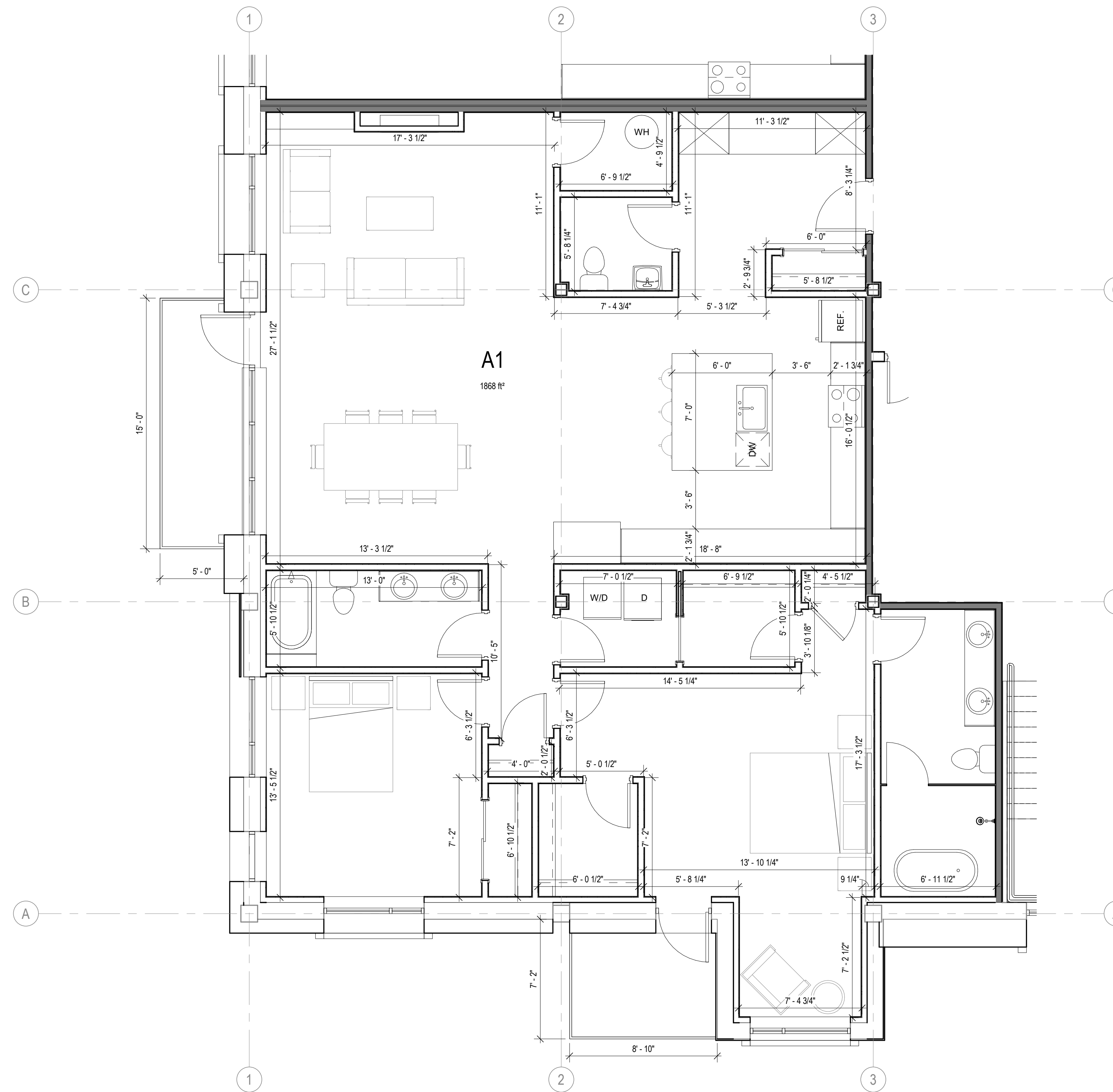
1 UNIT PLAN - A1 SCALE: 1/4" = 1'-0"
